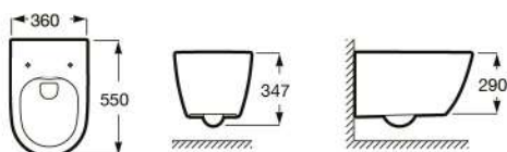
ONA 歐那掛牆馬桶
