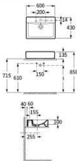
DIVERTA 碟塔檯上式面盆 方形
