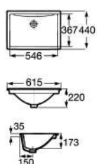
BERNA 貝娜檯下式面盆
