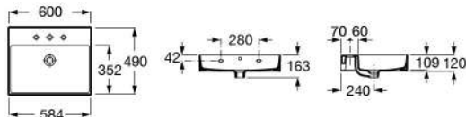
INSPIRA 英佩拉一體式面盆, 600mm
