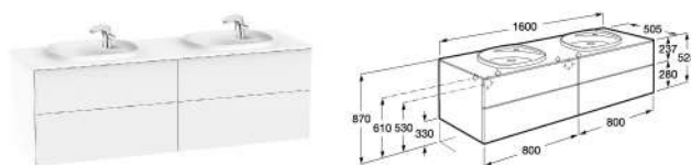
BEYOND 博越一體式雙面盆浴櫃
