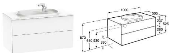
BEYOND 博越一體式面盆浴櫃
