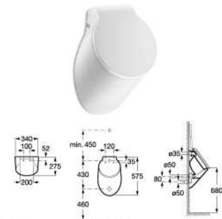
SPUN 斯賓小便斗連蓋
