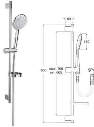
SENSUM ROUND 賽尚圓形蓮蓬頭伸降滑桿套裝組
