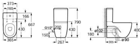
N-MERIDIAN 紐瑞分體馬桶水箱
