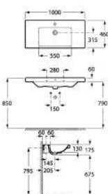
VICTORIA 維多利亞掛牆式面盆
